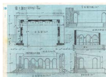
舞台（司令台）結構圖（陳孟和 繪）
